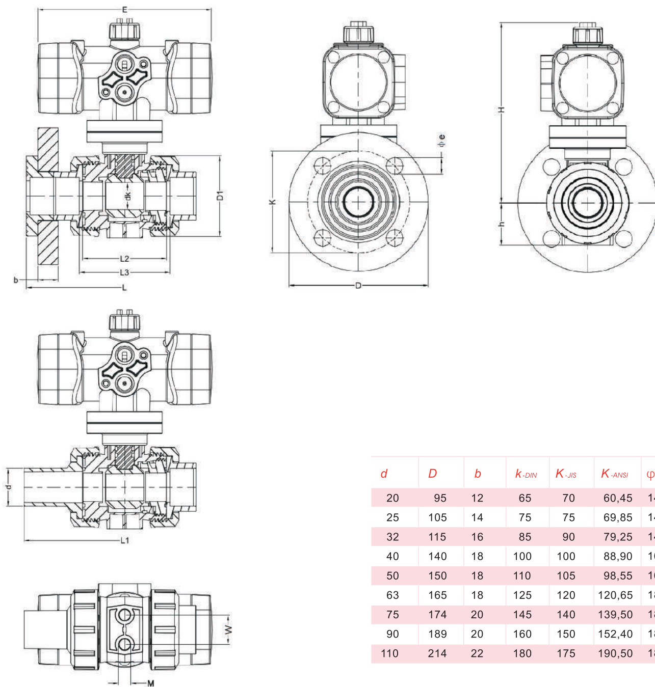
气动球阀尺寸数据
