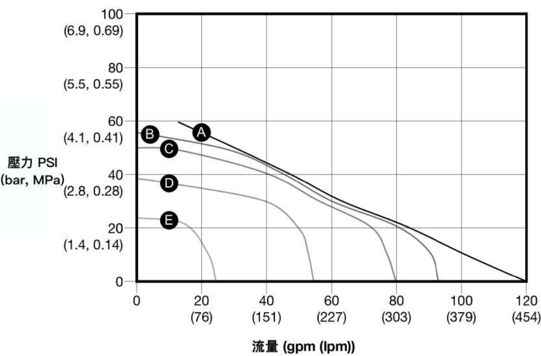
i120 (QTE) 球型性能表
