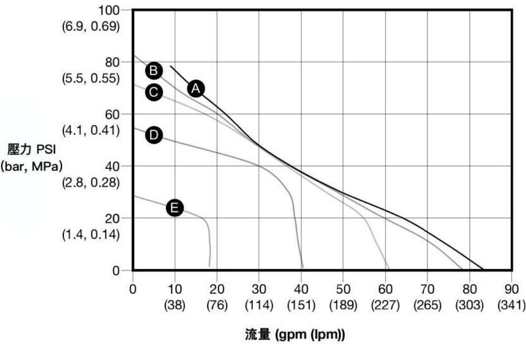
i120 (QTE) 球型性能表
