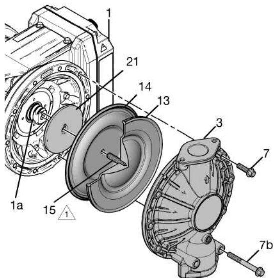
圖 23: 重新裝配超模壓隔膜
