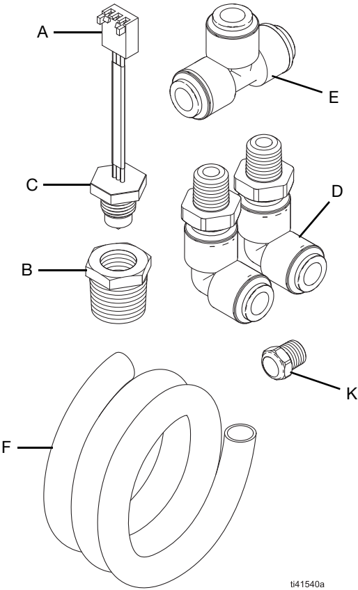
图 1：泄漏传感器配件包 25F108
