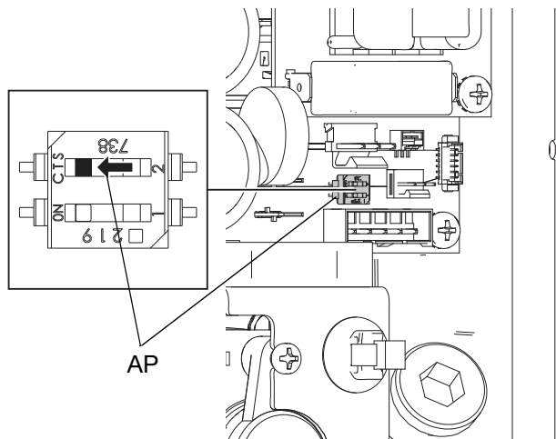
图 5：泄露传感器开关处于打开位置
