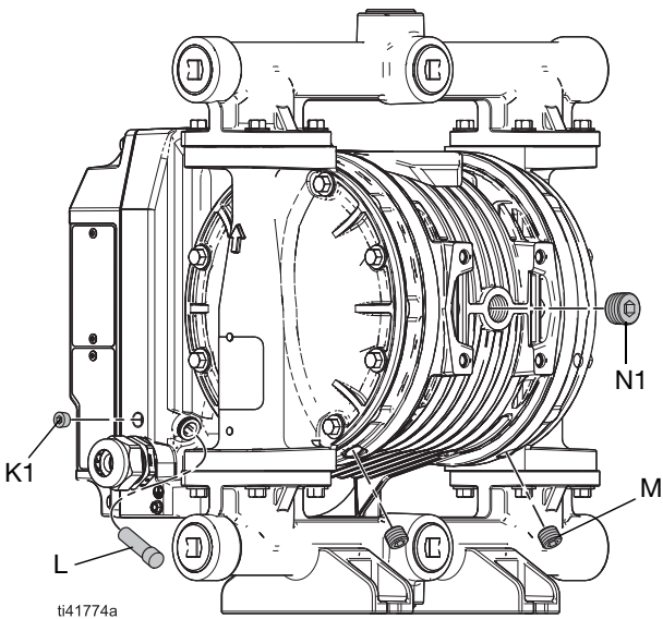
图 7：拆下插头，所示为工业型号
