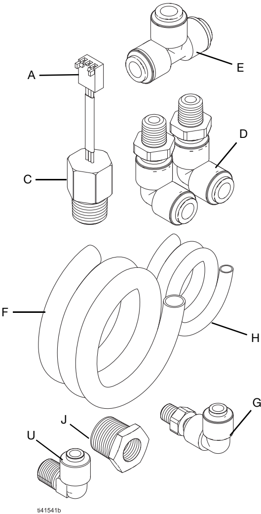
图 2：泄漏传感器配件包 25F109
