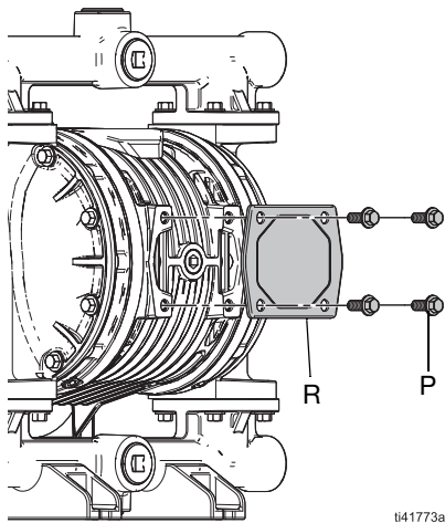
图 6：卸下紧固件和板，泵经认证仅可用于爆炸性环境或危险（分类）场所
